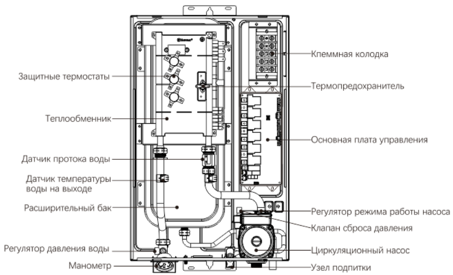
Рис. 2. Схема внутреннего устройства изделия
