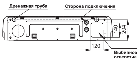
Положения соединений труб
